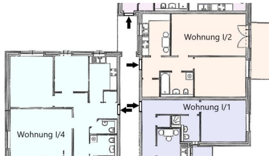
Grundriss 1
